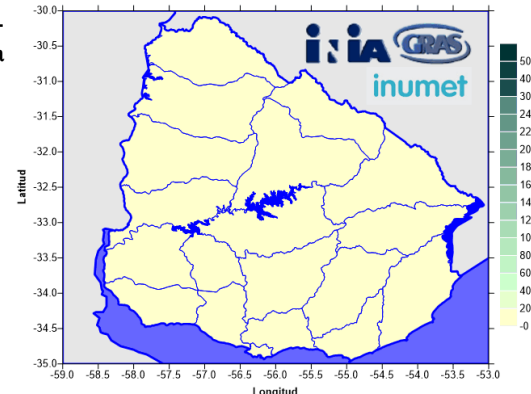
Agua no retenida acumulada (mm) en Febrero de 2018
