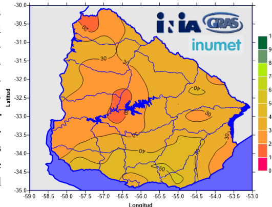
Índice de bienestar hídrico (%) Febrero de 2018
