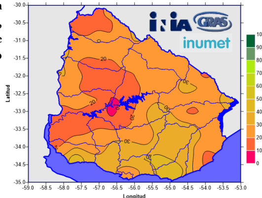
Porcentaje de agua disponible en el suelo Febrero de 2018
